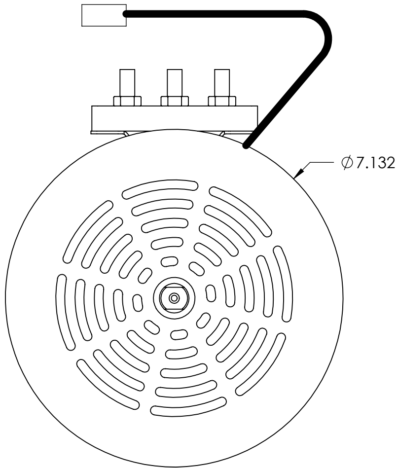
ENCODER END
