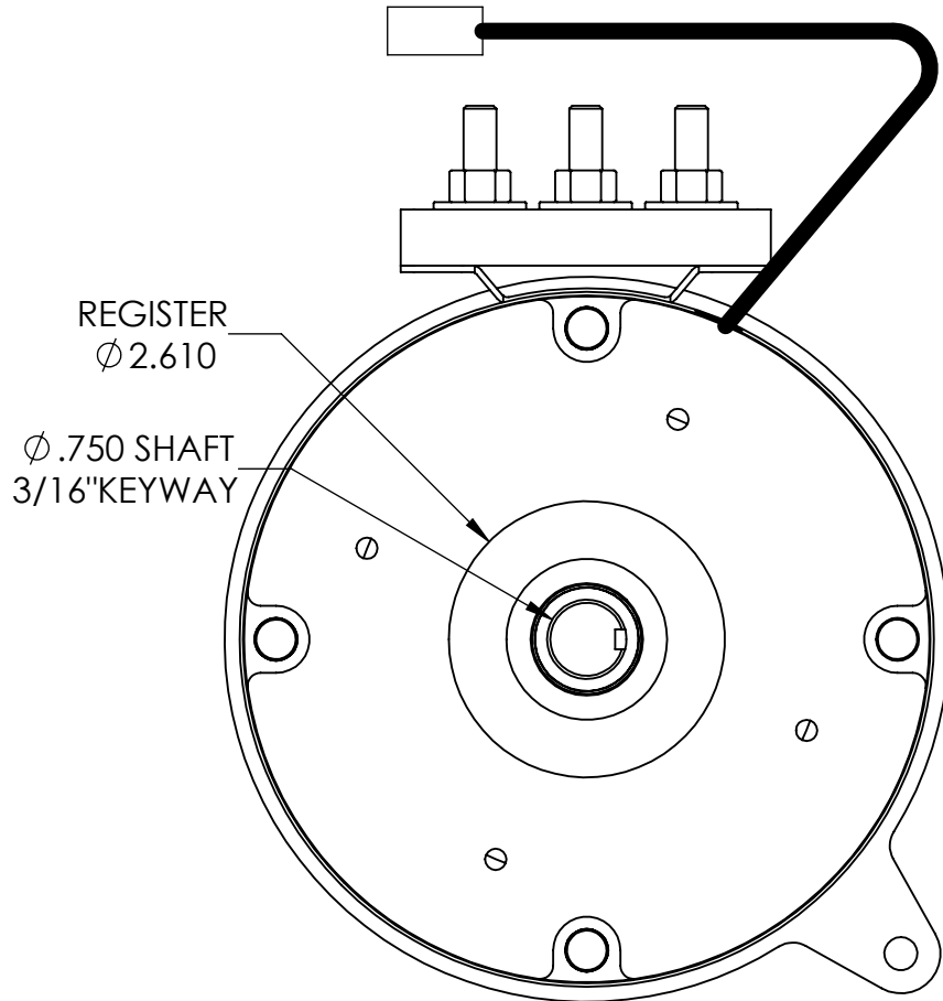
BRAKE END
