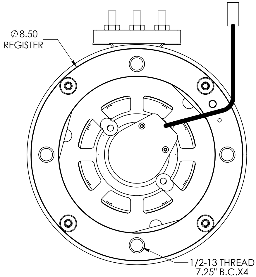
ENCODER END
