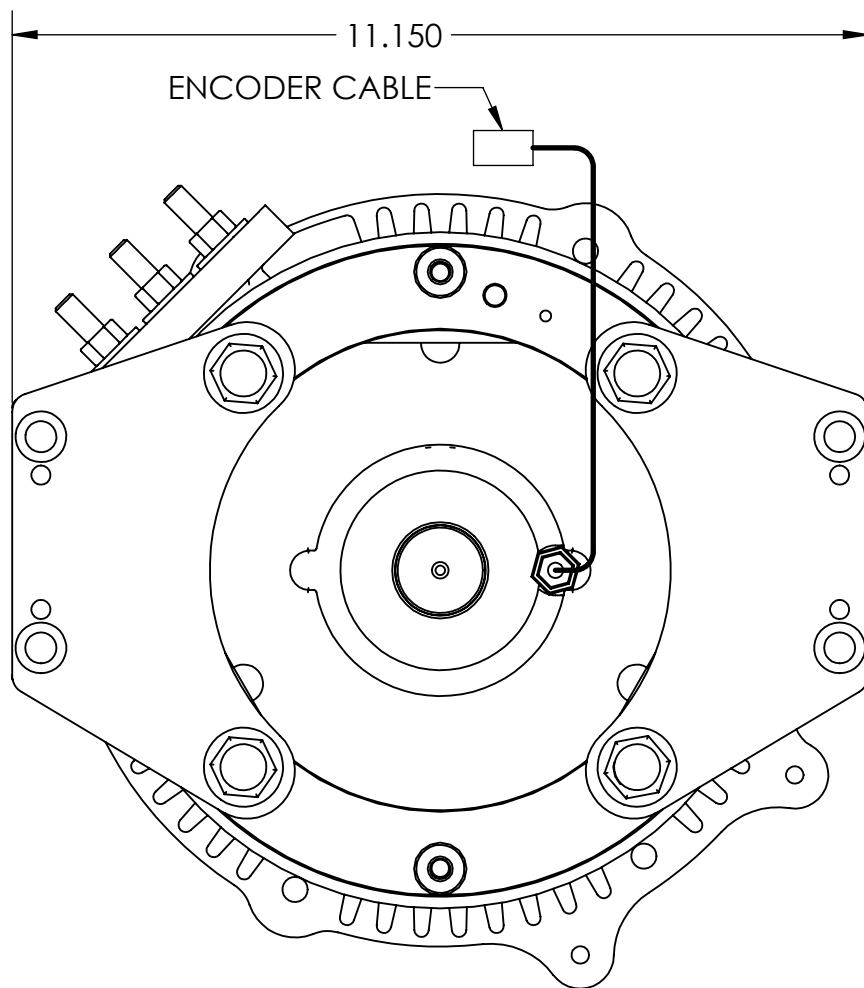
ENCODER END
